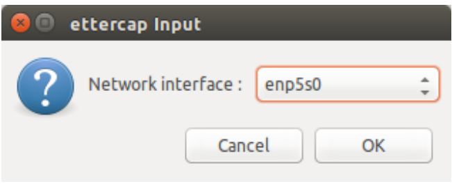
Выбор интерфейса
