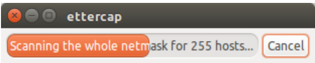
Сканирование хостов
